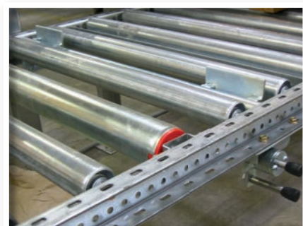
Butée escamotable manuelle
